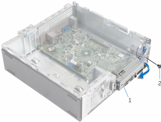
1 전면 패널
