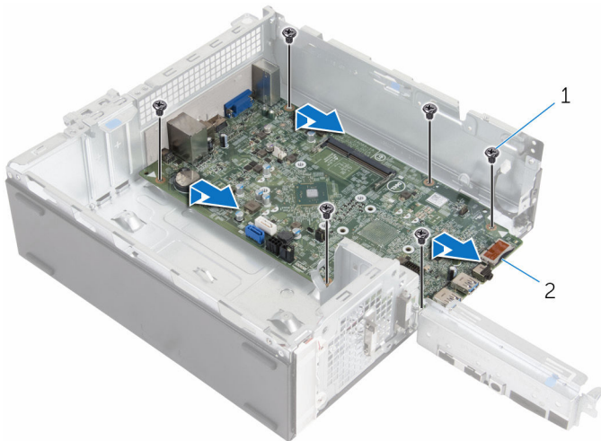
1 나사(6개)
